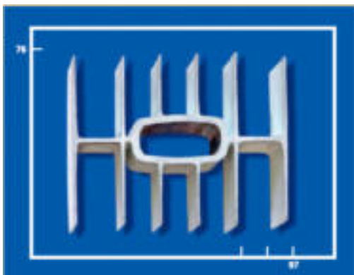
Поперечное сечение секции радиатора Seven 97 S 350/100; 500/100
